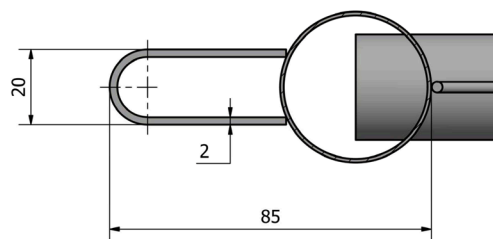
C-C ( 1:1 )
