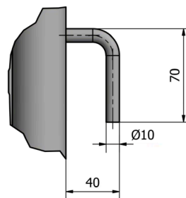
D ( 1:2 )
